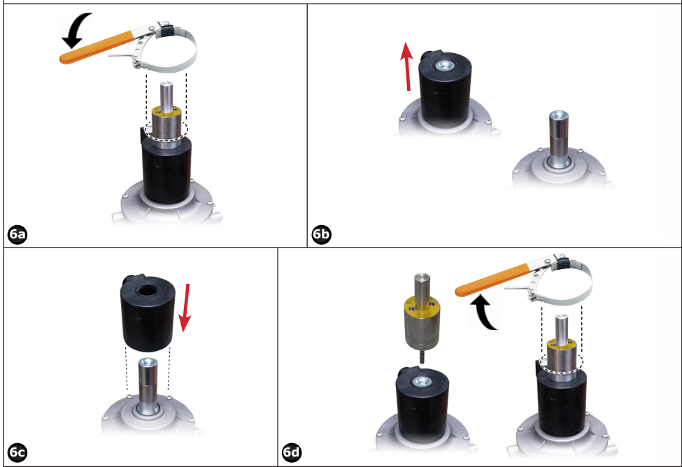
fig. 6 Sostituzione della bobina / Replacing the coil Remplacement de la bobine / Sustitución de la bobina
